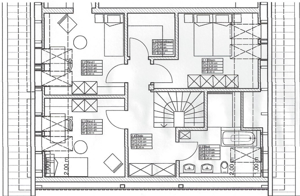
Obergeschoss
