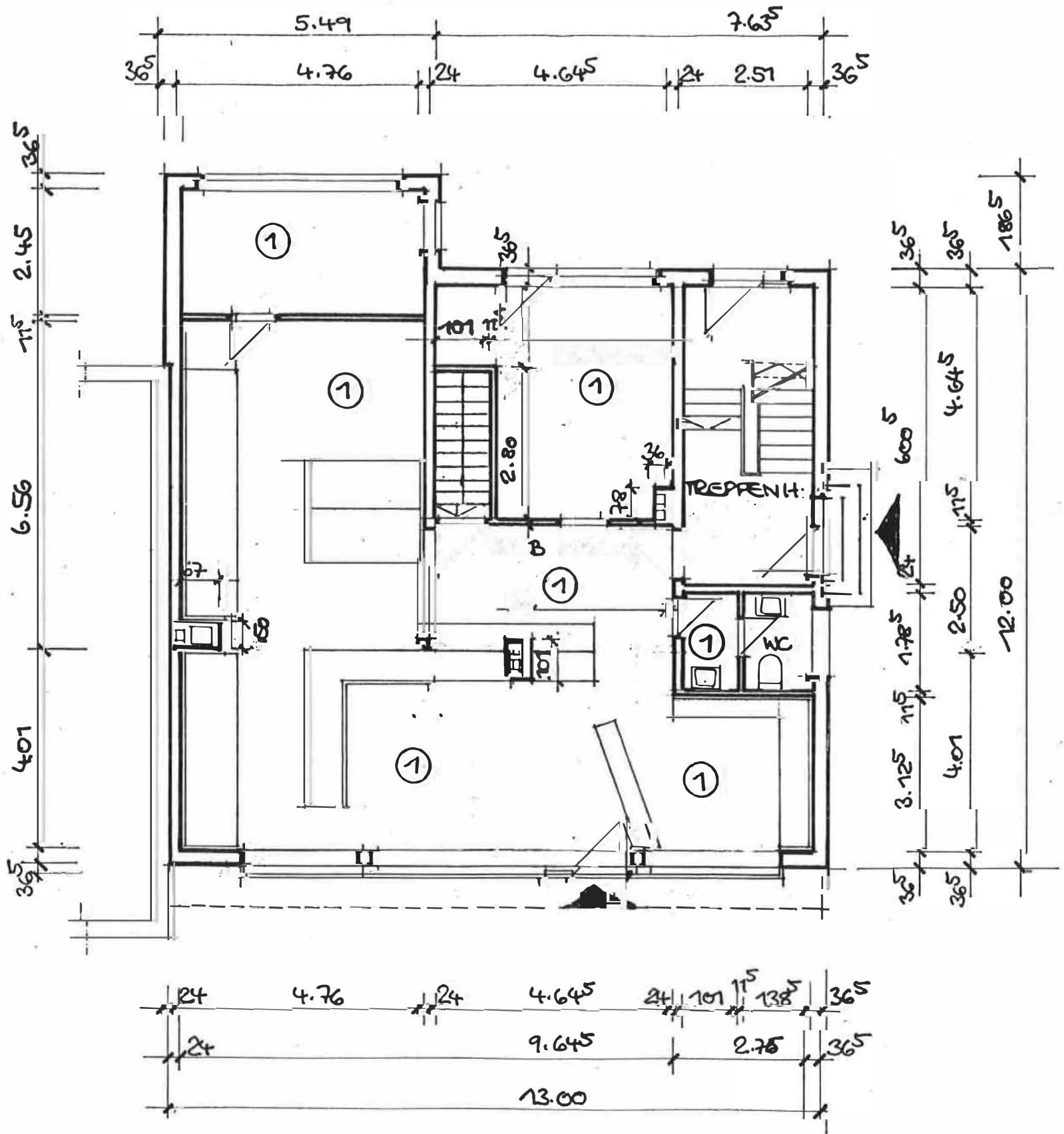
ERDGESCHOSS M.1:100
