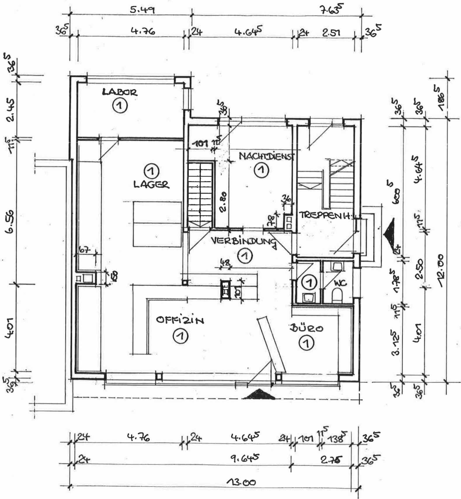
ERDGESCHOSS M.1:100
