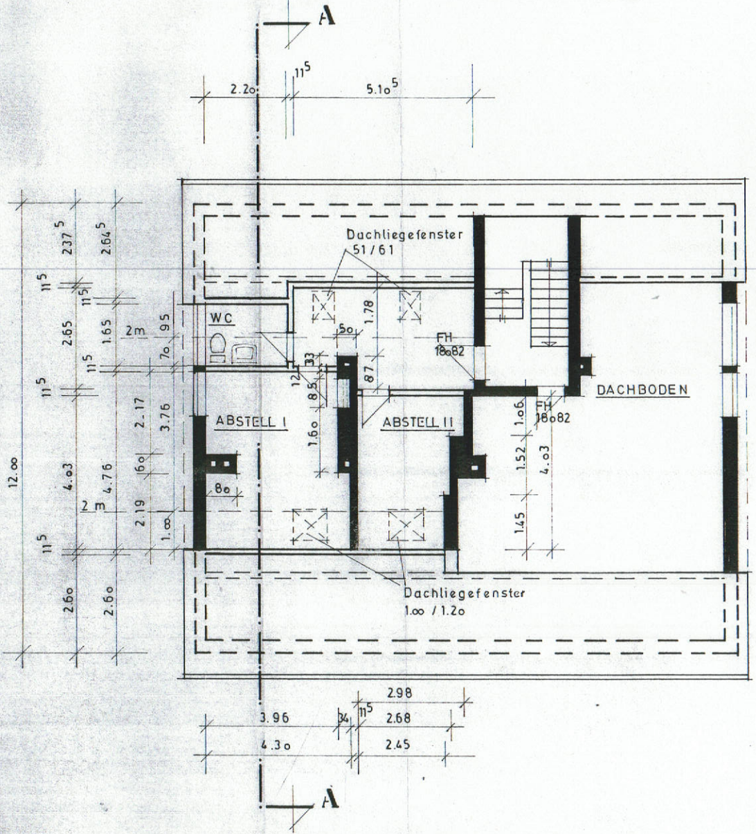
DACHGESCHOSS
