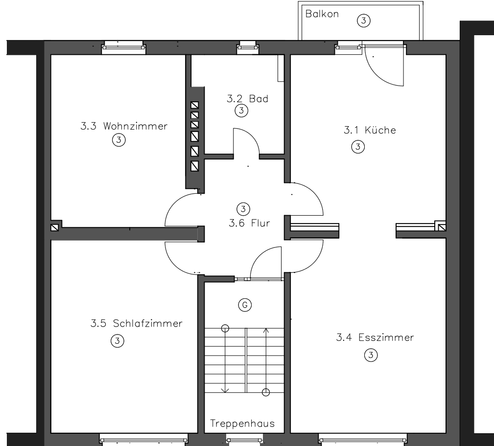
2.Obergeschoss Schulstraße 33 Münster
